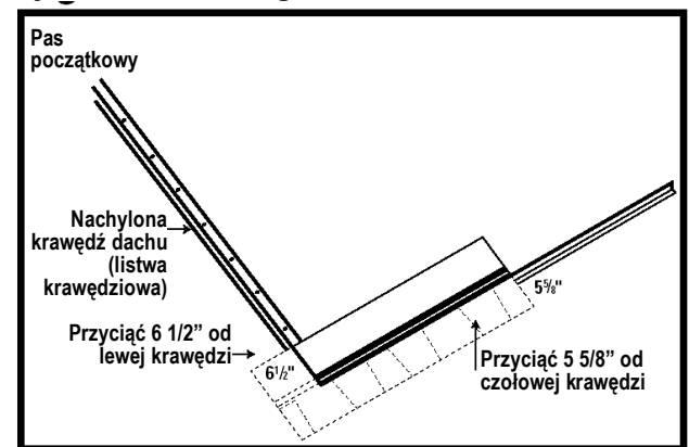
Rys. 5 Układanie gontów
