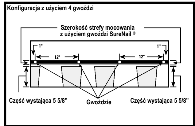
Rys. 4a Schemat mocowania gontów na dachu stromym lub mansardowym
